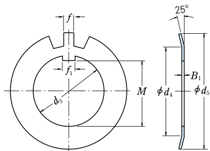
Straight-Tab
